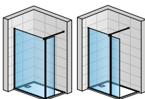
STR4P +BTE2 STR4P +BTE3
