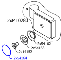
DET.B
